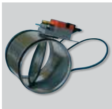
REMP Compuertas motorizadas proporcionales circulares con cuerpo de acero galvanizado y motorización controlada por sonda de CO 2 . El servomotor funciona proporcionalmente a la señal 0-10V enviada por la sonda. Intercalando el módulo BEAS se pueden ajustar las posiciones de apertura mínima y máxima. Se utilizan en los sistemas de ventilación multizona tipo proporcional.
